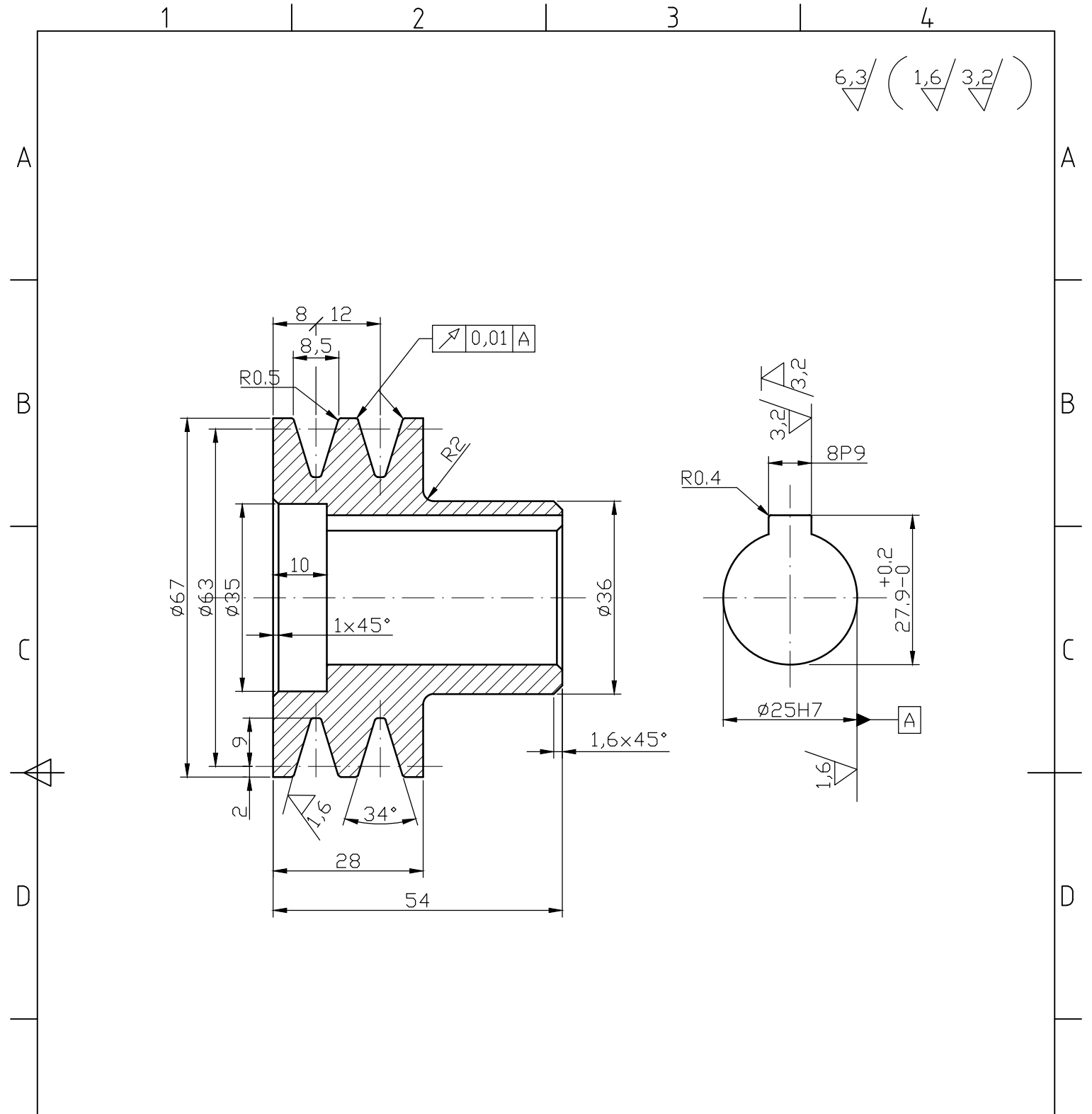
Věncový řemenice 63-SPZ-2 ČSN 02 3180
